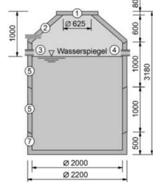
Zisternen mit 9,5 m 3 Volumen
