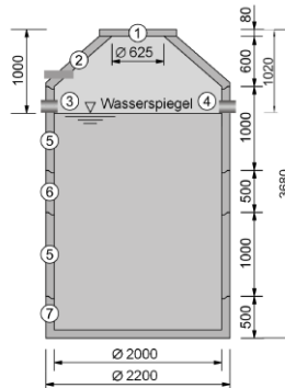
Zisternen mit 8,0 m 3 Volumen
