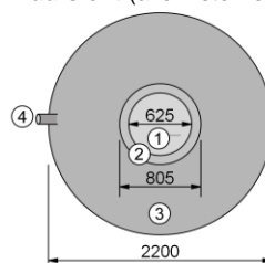
Draufsicht (alle Zisternen)
