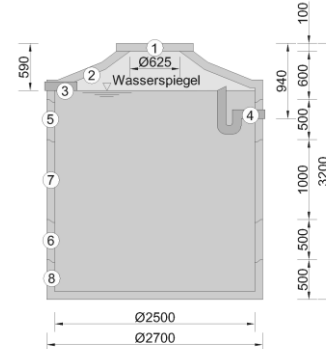
Zisternen mit 12,3 m 3 Volumen
