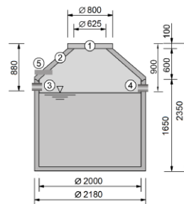
Maßbild Zisterne mit 4,0 m³ Volumen
