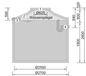
Zisterne mit 9,3 m³ Volumen
