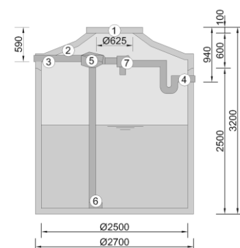
Maßbild Zisterne mit 11,8 m³ Volumen
