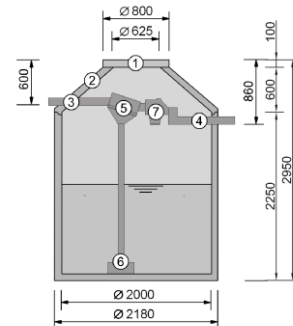
Maßbild Zisterne mit 6 m³ Volumen
