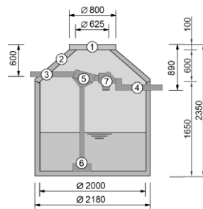
Maßbild Zisterne mit 4,0 m³ Volumen
