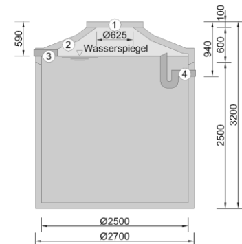
Zisterne mit 11,8 m³ Volumen
