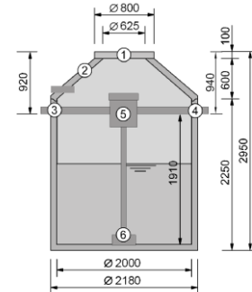
Maßbild Zisterne mit 6 m³ Volumen
