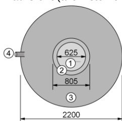
Draufsicht (alle Zisternen)
