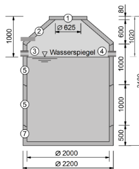
Zisternen mit 9,5 m³ Volumen
