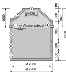
Zisternen mit 5,0 m³ Volumen
