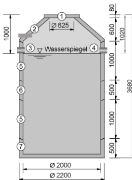
Zisternen mit 8,0 m³ Volumen
