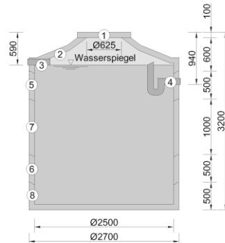
Zisternen mit 12,3 m³ Volumen
