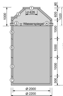
Zisternen mit 9,5 m³ Volumen
